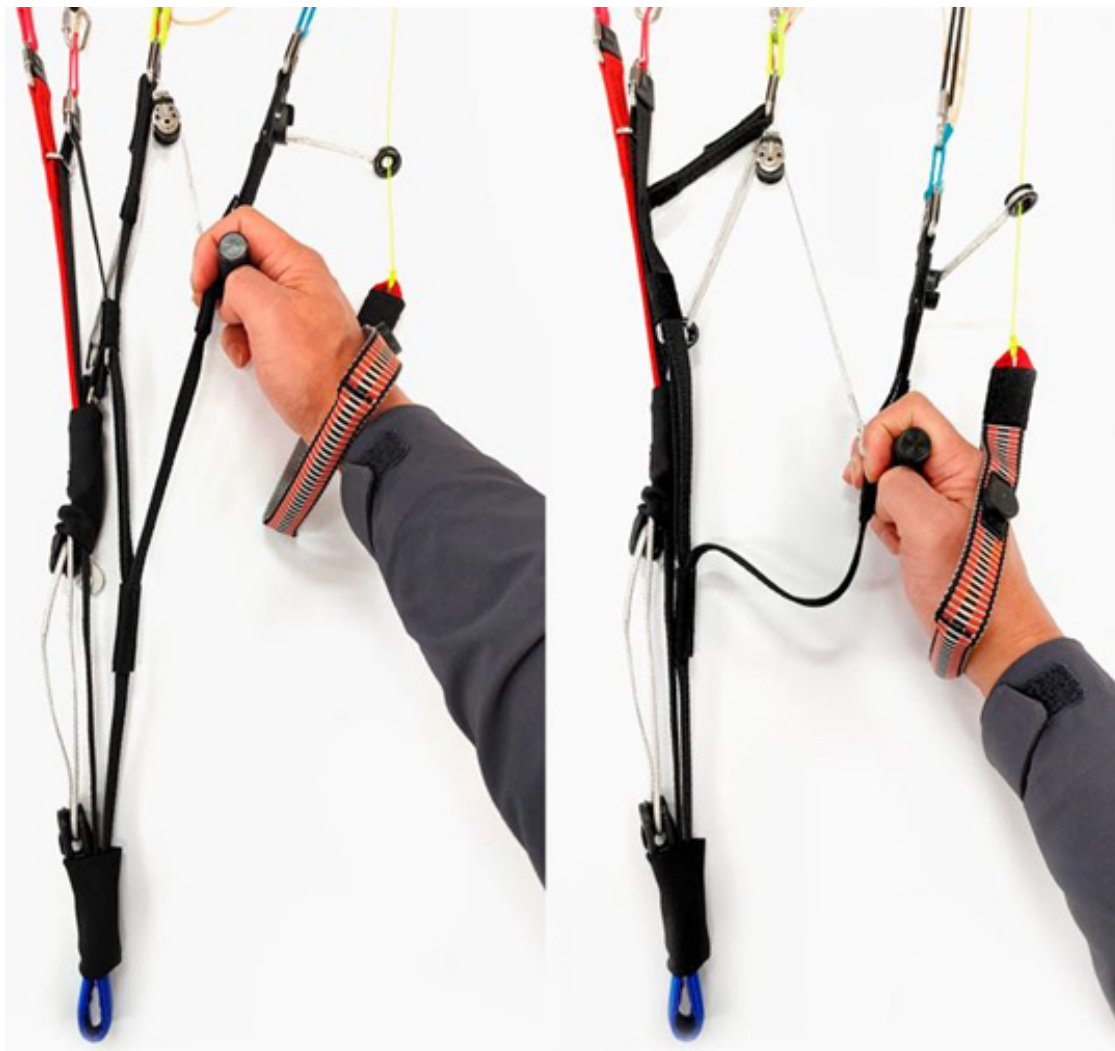
Illustration : Comment attraper et tirer l'élévateur SMART de l'Evora
