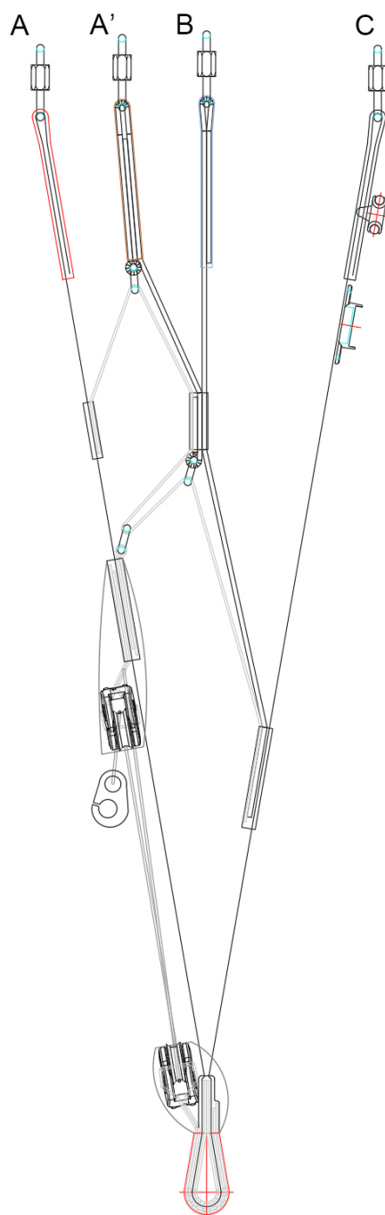
Illustration : élévateurs Evora (standard)
