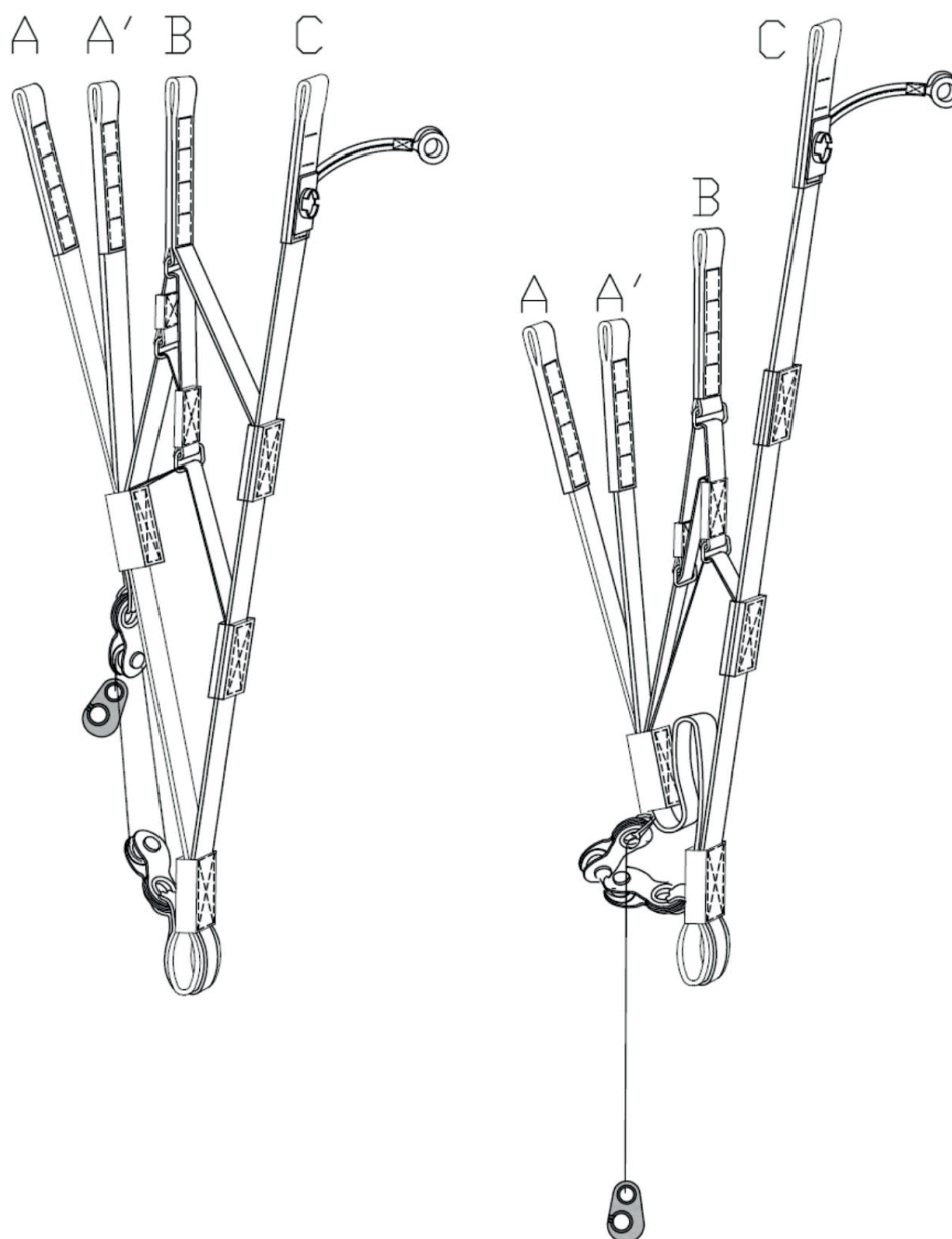
Illustration : élévateurs Calypso
