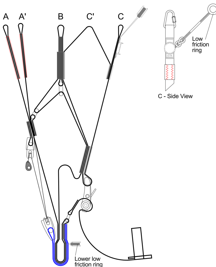
Illustration : élévateurs Pegasus 4
