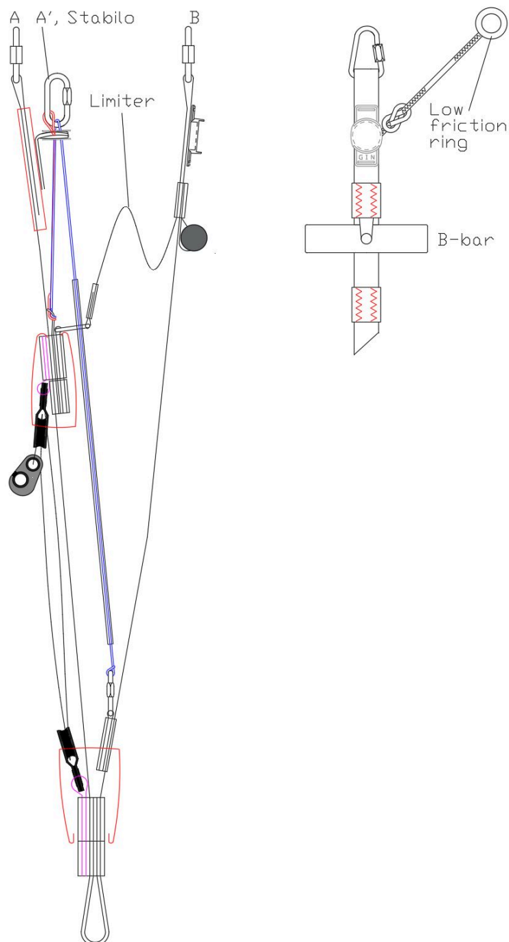
Abbildung: Camino 2 Tragegurt
